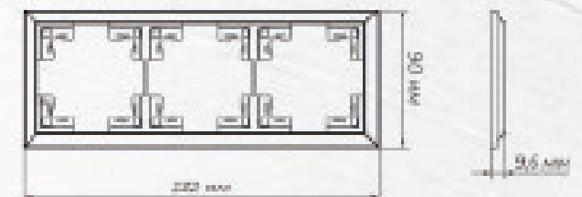
Тримісна
