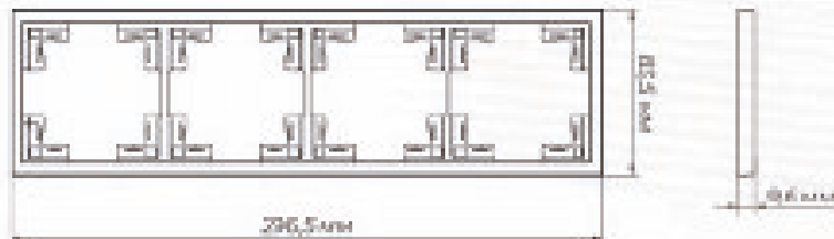
Чотиримісна
