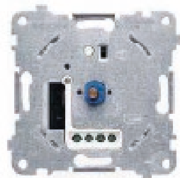
Механізм димера 250W (Smart WiFi)
