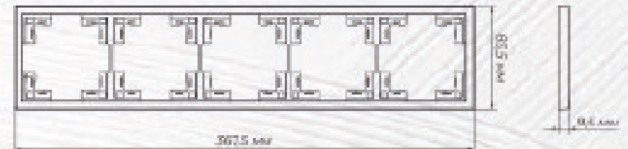
П'ятимісна
