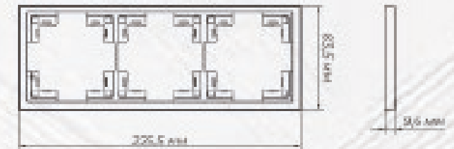
Тримісна
